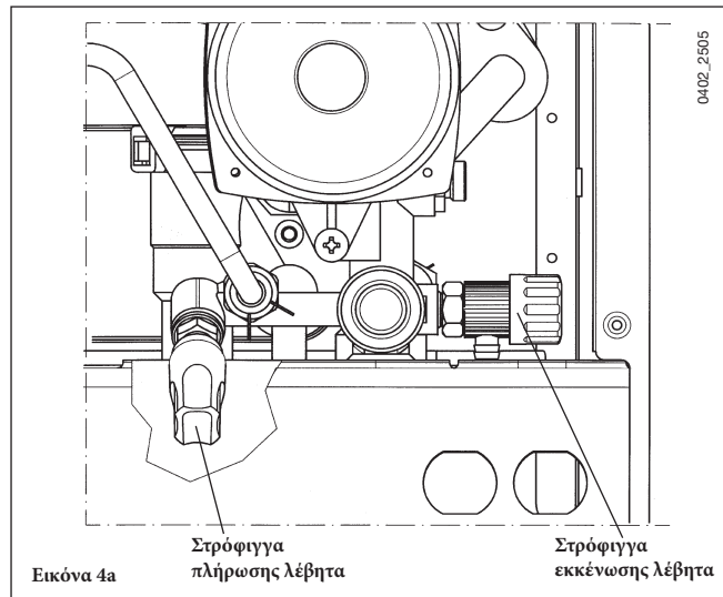
STAR CONDENS 240 - 280
