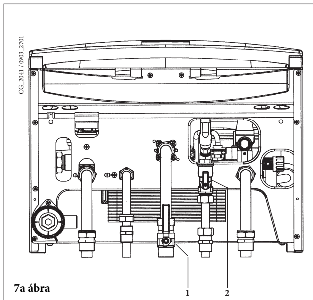
STAR CONDENS 240 - 280
